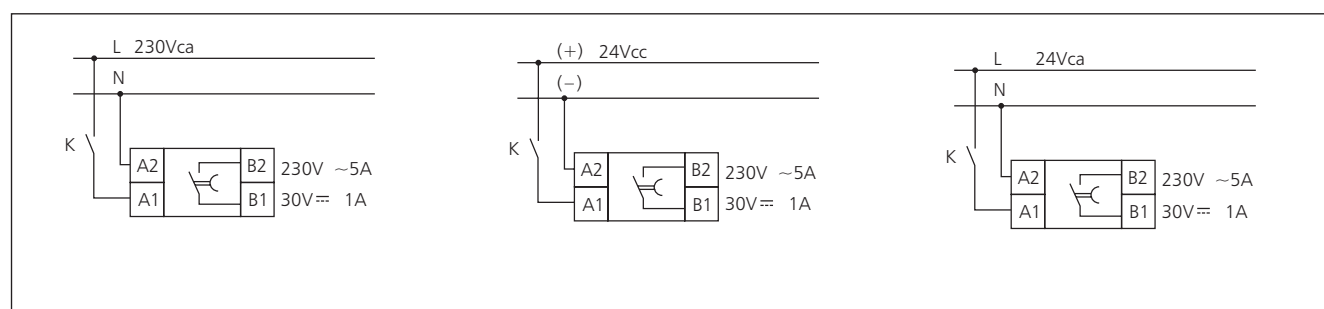
Esquema de conexiones del temporizador NTE8-B
