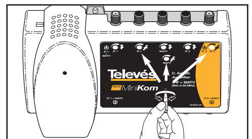
Ajuste de pendiente de salida / Ajuste do pendente de saída / Ajustement du pente de sortie / Output slope signal variation / Regolazione pendenza in uscita
