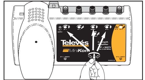
Ajuste del nivel de salida / Ajuste do nivel de saída / Ajustement du niveau de sortie / Output signal variation / Regolazione livello di uscita
